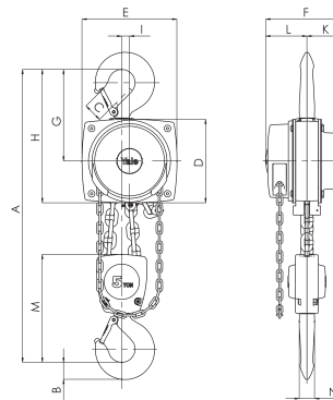
Yalelift 360, 5000 kg, double fall
