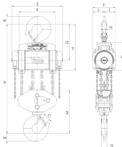
Yalelift 360, 20000 kg, six falls
